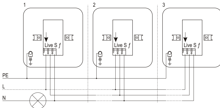
Elektrooniliste moodulite ühendusskeem koos valgusregulaatoriga IŠR-003 ja IŠR-003-01
