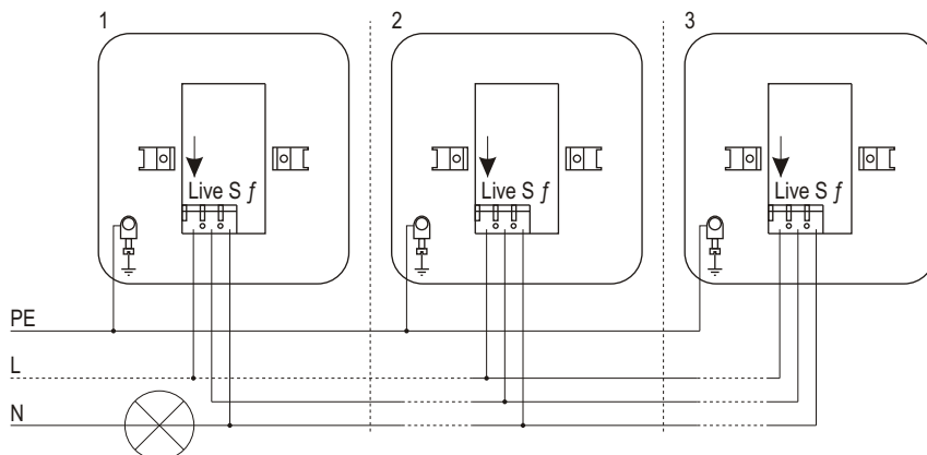
Elektronisko moduļu pieslēgšanas shēma kopā ar gaismas regulatoru IŠR-003 un IŠR-003-01
