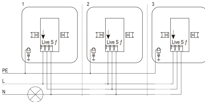
Elektroninių modulių pajungimo schema kartu su šviesos reguliatoriumi IŠR-003 ir IŠR-003-01
