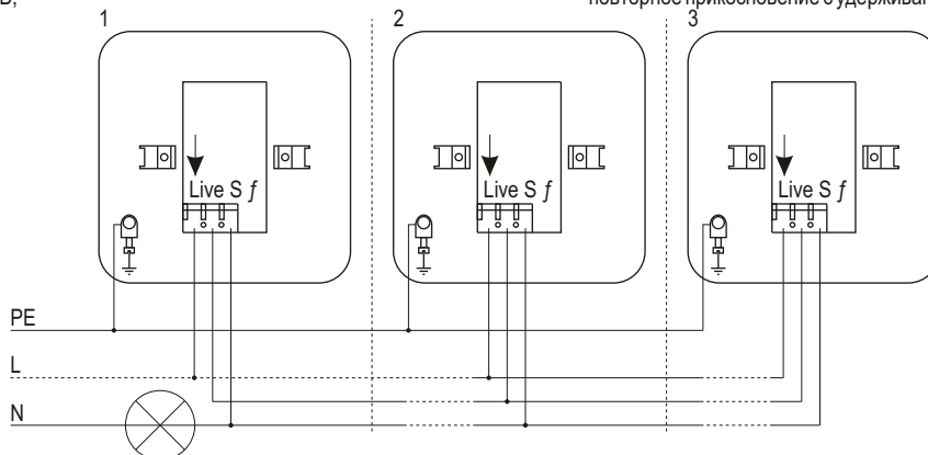
Схема присоединения электронных модулей совместно с регуляторами света IŠR-003 и IŠR-003-01
