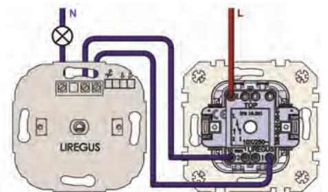
Šviesos srauto reguliatorius, su 1 kl. perjungikliu
